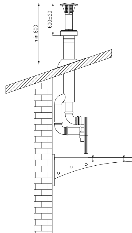
Рис.28.: Тип C32
