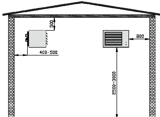
Рис. 14.: Минимальные защитные расстояния
