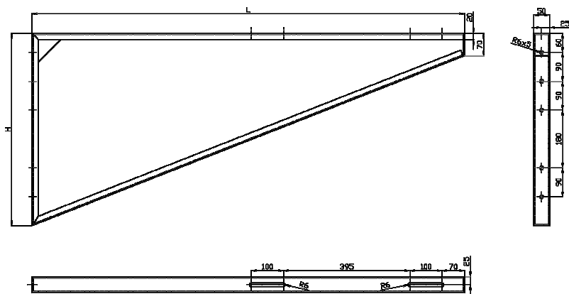
Рис. 17: Размеры консоли
